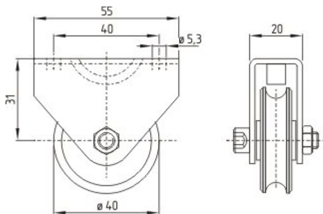
Rysunek wymiarowy (inne)
