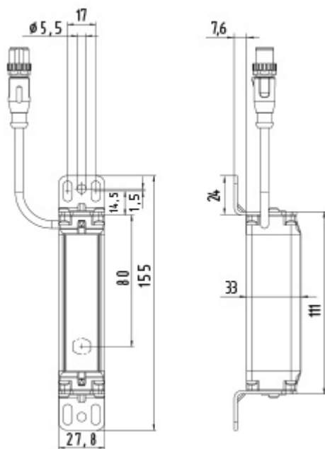
Rysunek wymiarowy (element podstawowy)
