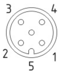
Układ zestyków
