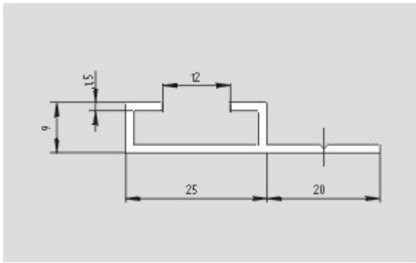
Rysunek wymiarowy (element podstawowy)
