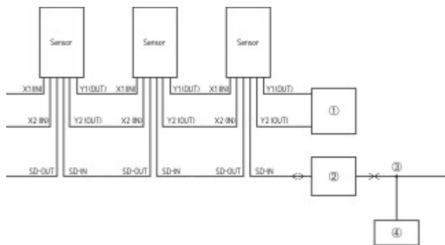
Przykład okablowania
