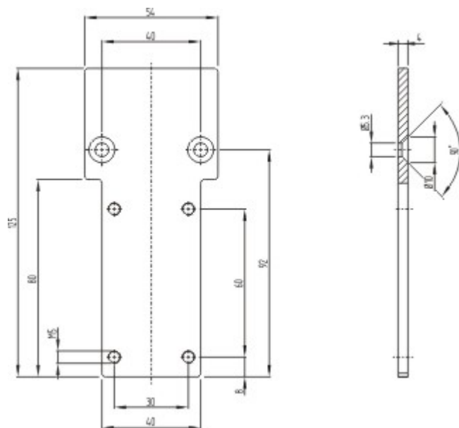
Rysunek wymiarowy (element podstawowy)
