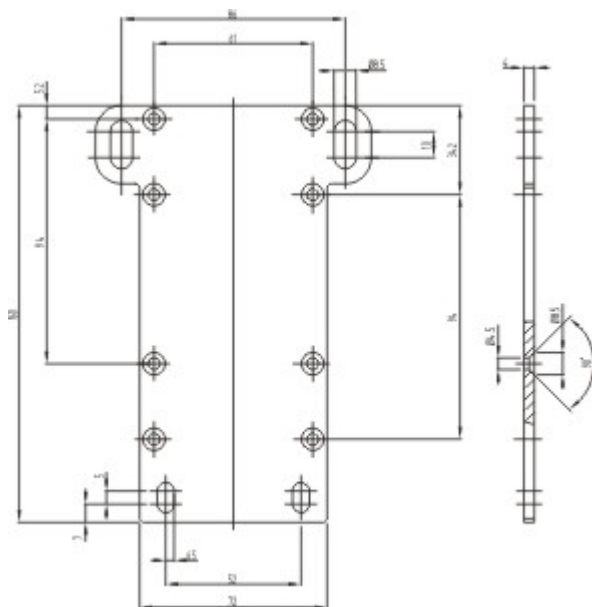
Rysunek wymiarowy (element podstawowy)
