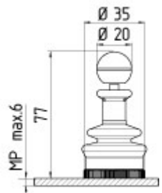
Rysunek wymiarowy (inne)
