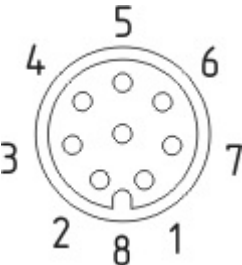
Układ zestyków
