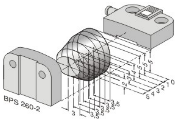
Krzywa charakterystyczna
