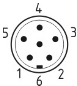
Układ zestyków
