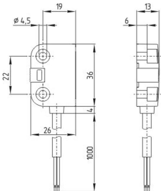
Rysunek wymiarowy (element podstawowy)
