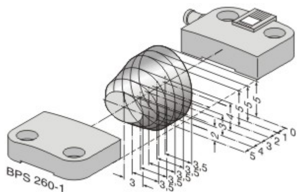
Krzywa charakterystyczna
