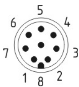
Układ zestyków
