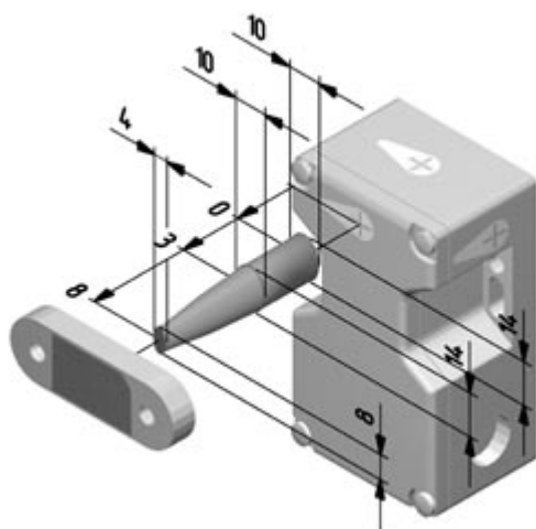
Rysunek wymiarowy (inne)
