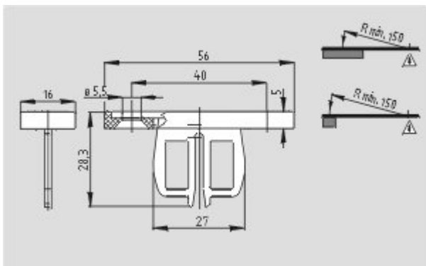
Rysunek wymiarowy (aktywator)
