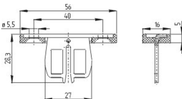
Rysunek wymiarowy (inne)
