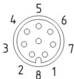
Układ zestyków
