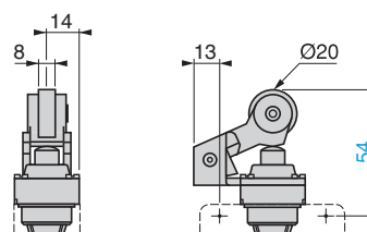
ZCK D219, D239
